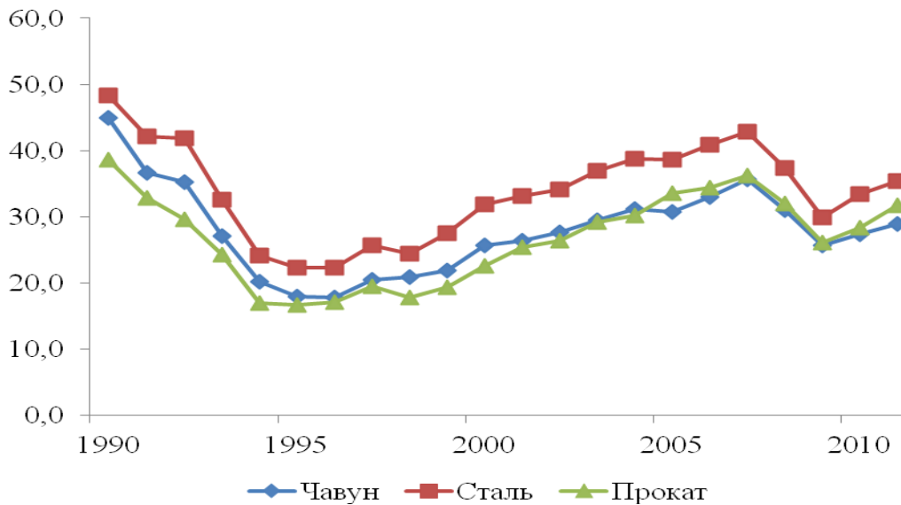
Рис. 1. Виробництво основних видів металопродукції в Україні в 1990-2011 рр. (млн. т)
